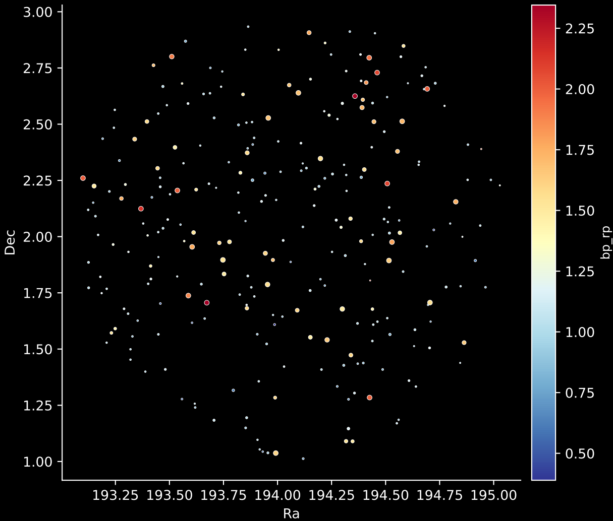
GALAH DR4 Field: [9273] Stars: 269
