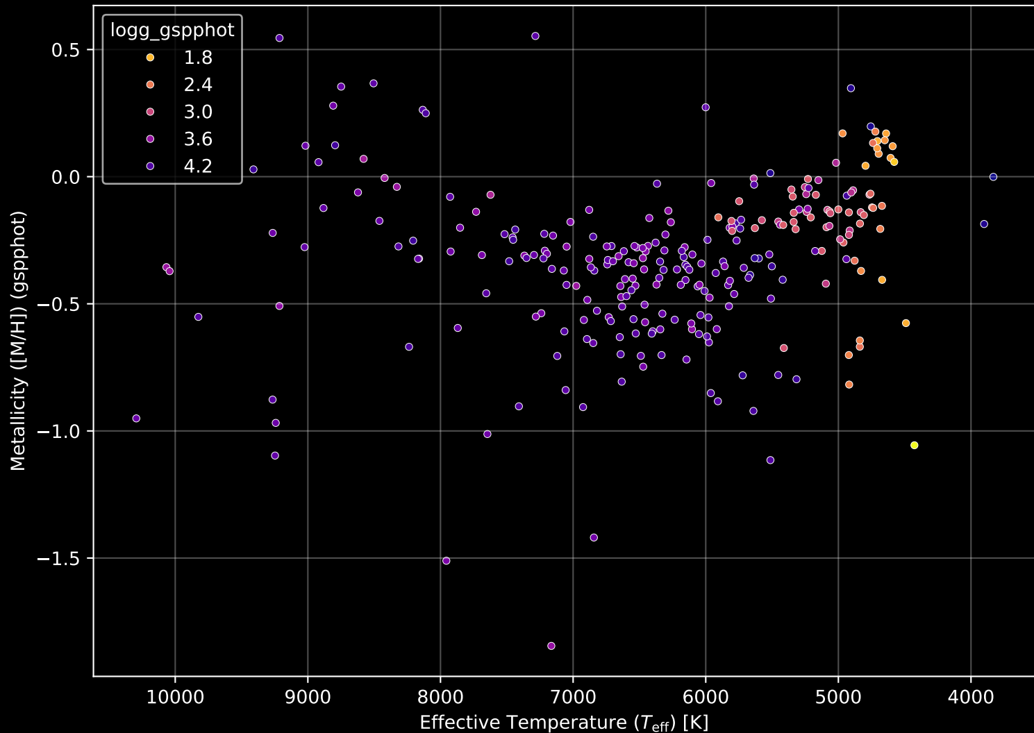
GALAH DR4 Field: [9273] Stellar Population Parameters (n= 269)
