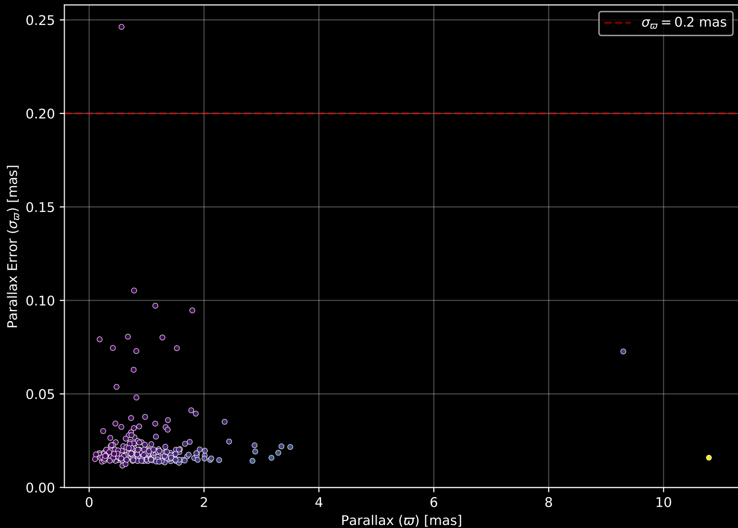
GALAH DR4 Field: [9273] Parallax Quality (n= 269)
